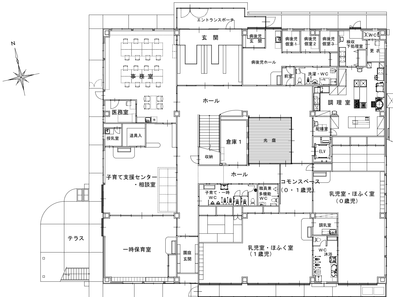
1 階 平 面 図
