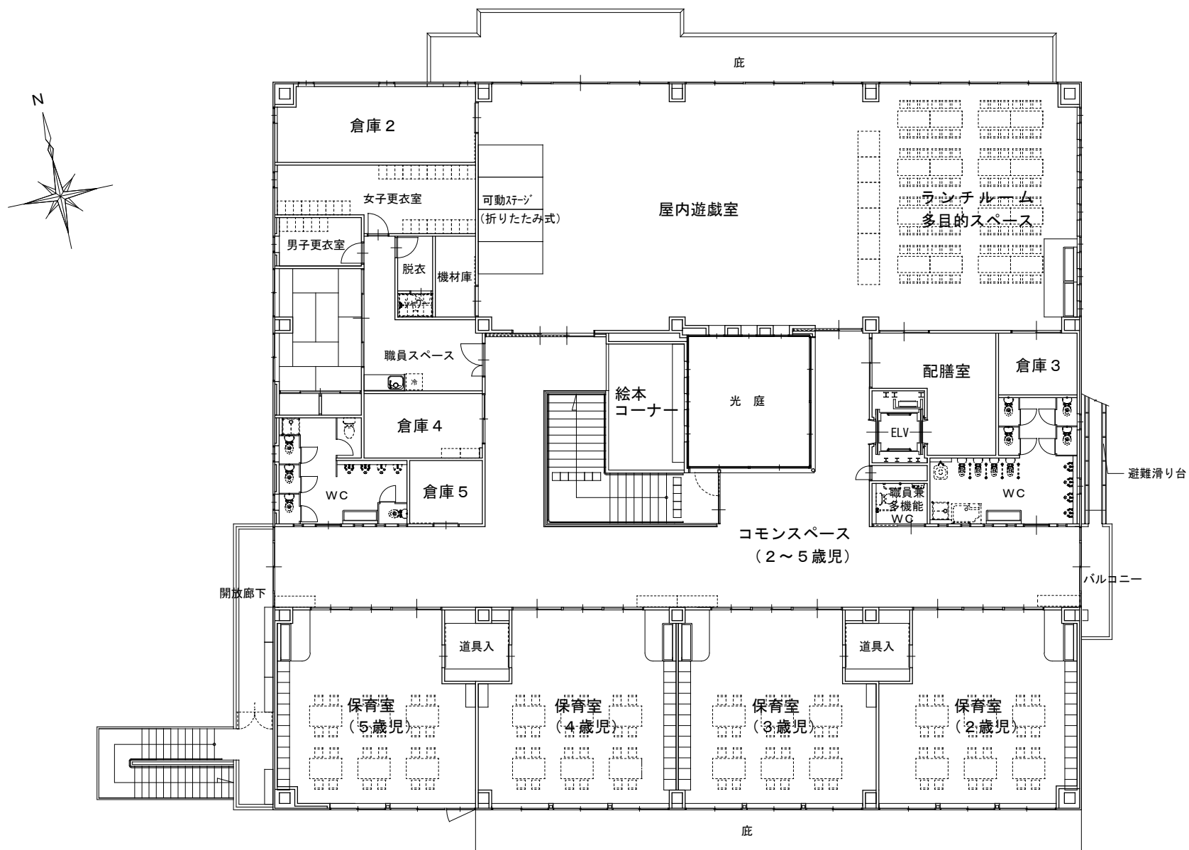
2 階 平 面 図
