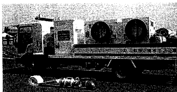
ポンプ6台を稼働する排水ポンプ車
