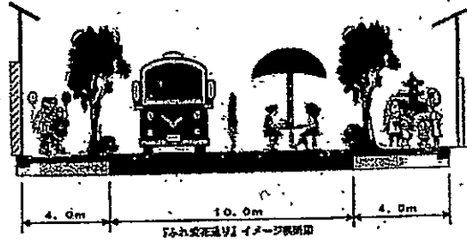
社会実験実施時の断面イメージ
