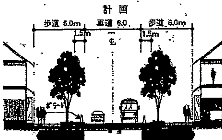
整備前後の道路横断構成の比較
