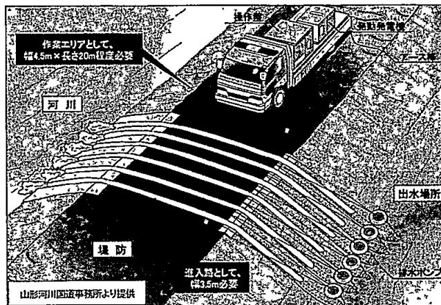
「排水ポンプ車ののはたらき」
