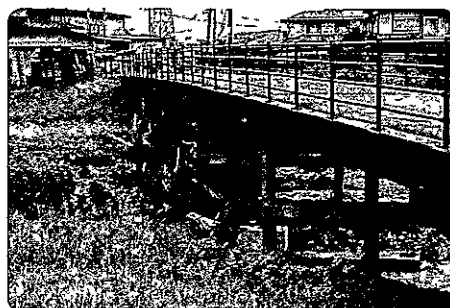
【谷柏橋(本沢川)】流木詰まりで流れが膨らみ、児童遊園側の土地がえぐられる
