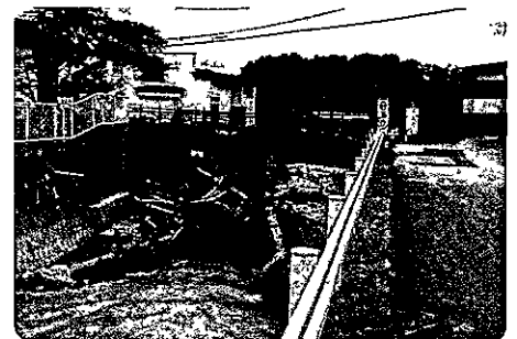
【本沢橋(本沢川)】流木が引っかかり欄干が崩壊
