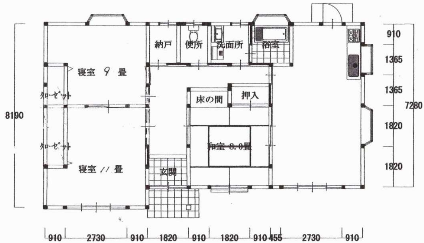
1 階平面図
